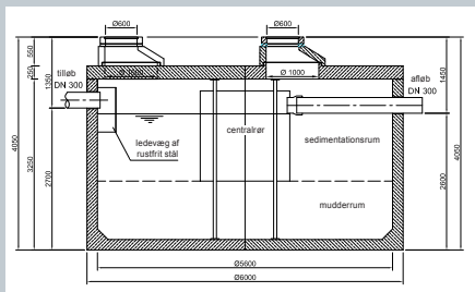
ENREGIS/Sedimentationsanlæg MSA 5600
