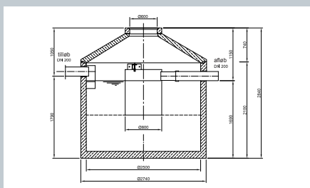
ENREGIS/Sedimentationsanlæg MSA 2500 N
